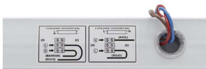
CONEXIÓN 1 EXTREMO CONEXIÓN 2 EXTREMOS
